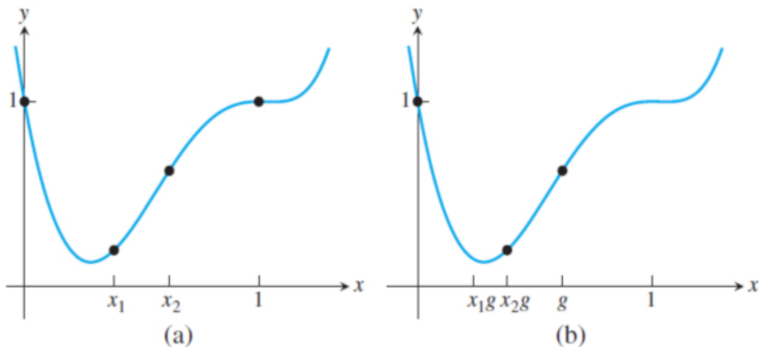
Figura 5: Căutarea secțiunii de aur. (a) Evaluăm funcția obiectiv în două puncte x_1, x_2 din intervalul curent [0, 1] . Dacă f(x_1) \leq f(x_2) , atunci noul interval va fi [0, x_2] . (b) În pasul următor, luăm g = x_2 și repetăm aceeași comparație cu x_1g și x_2g .
