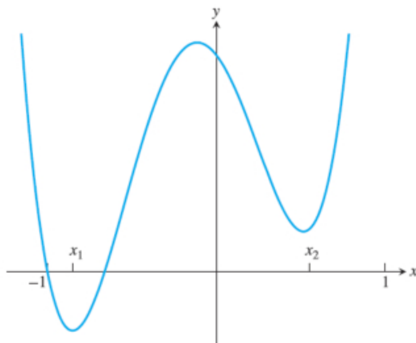
Figura 4: Problema de minimizare pentru
