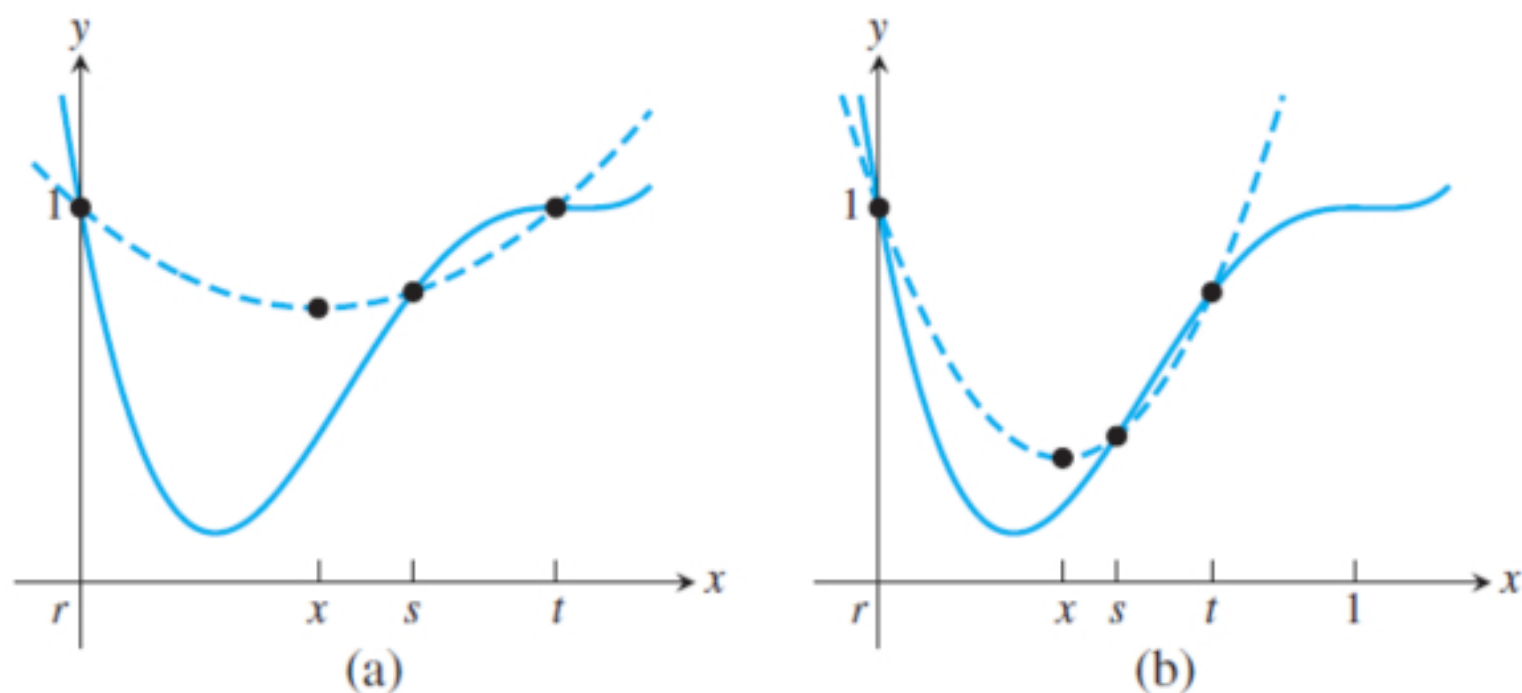
Figura 7: Interpolarea parabolică succesivă. (a) O parabolă este desenată prin cele trei puncte curenți r , s , t , și minimul x al parabolei este folosit pentru a înlocui valoarea curentă a lui s . (b) Pasul este repetat cu noile puncte r , s , t .
